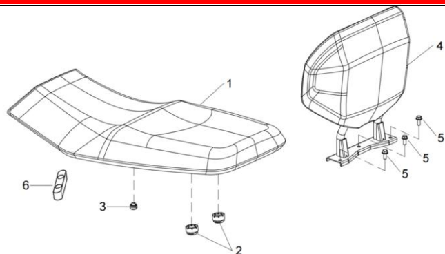
DIAGRAMMA 2025 SEDILI AODES F13
