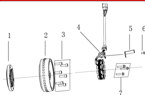
DIAGRAMMA 2025 ASSEMBLAGGIO MAGNETO AODES E06
