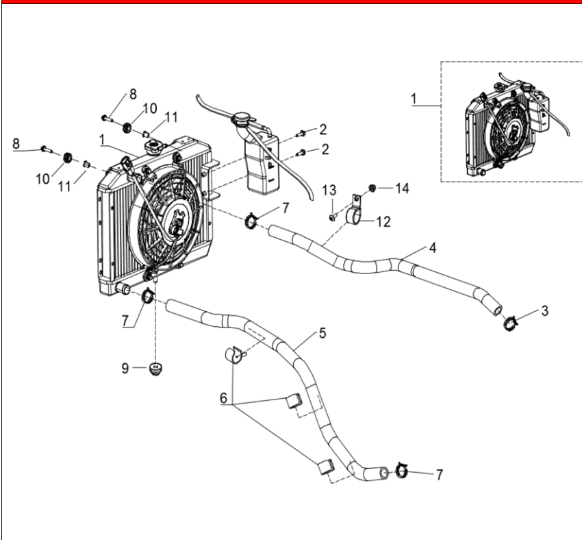
DIAGRAMMA 2025 SISTEMA DI RAFFREDDAMENTO AODES F14
