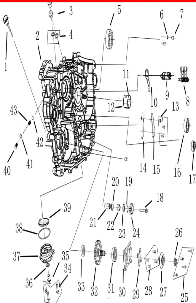
DIAGRAMMA 2025 CARTER SINISTRO B AODES E10
