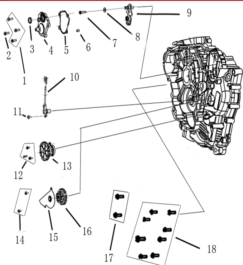
DIAGRAMMA 2025 CARTER SINISTRO AODES E09
