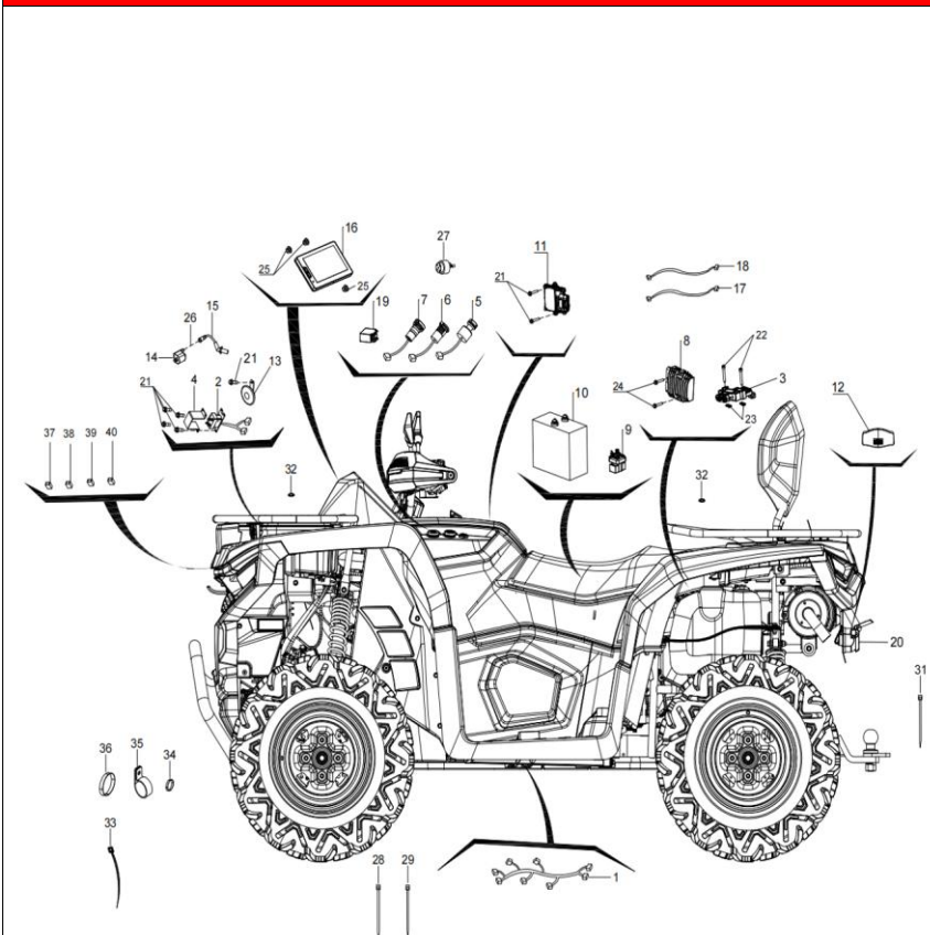
DIAGRAMMA 2025 PARTI ELETTRICHE AODES F15
