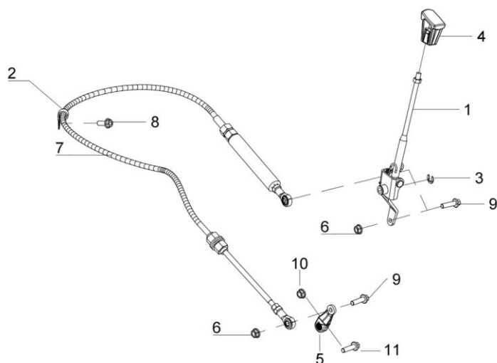
DIAGRAMMA 2025 SISTEMA DI CAMBIO AODES F21
