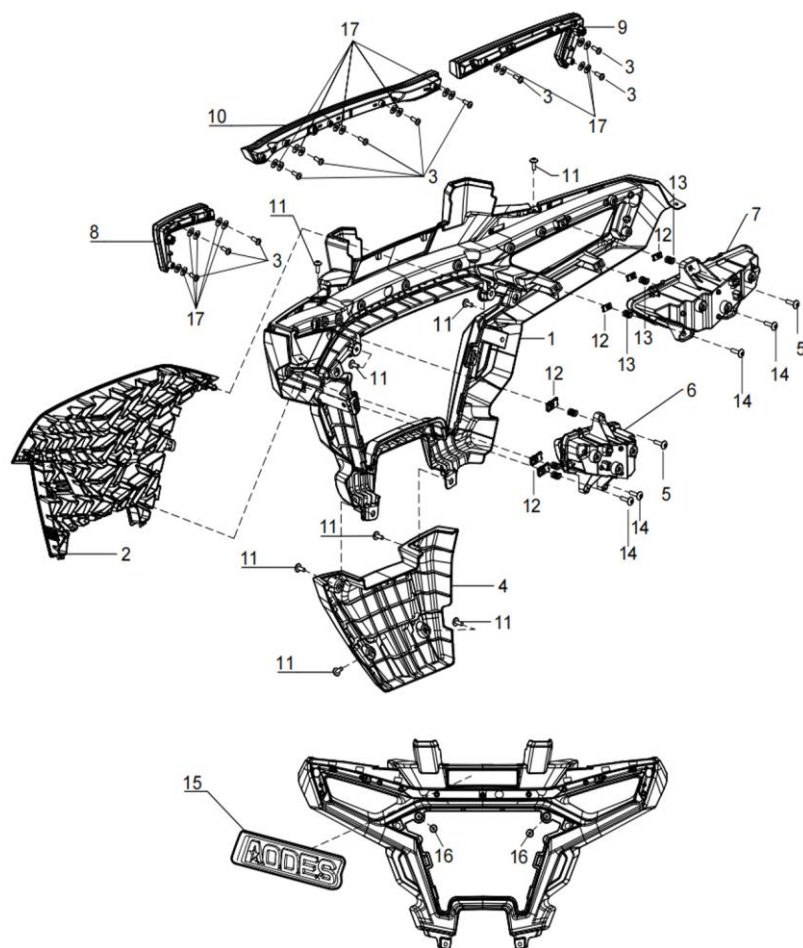
DIAGRAMMA 2025 PLASTICA ANTERIORE-2 AODES F17
