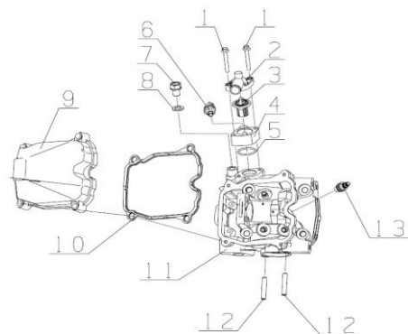
DIAGRAMMA 2025 COMPONENTI TESTA CILINDRO AODES E01
