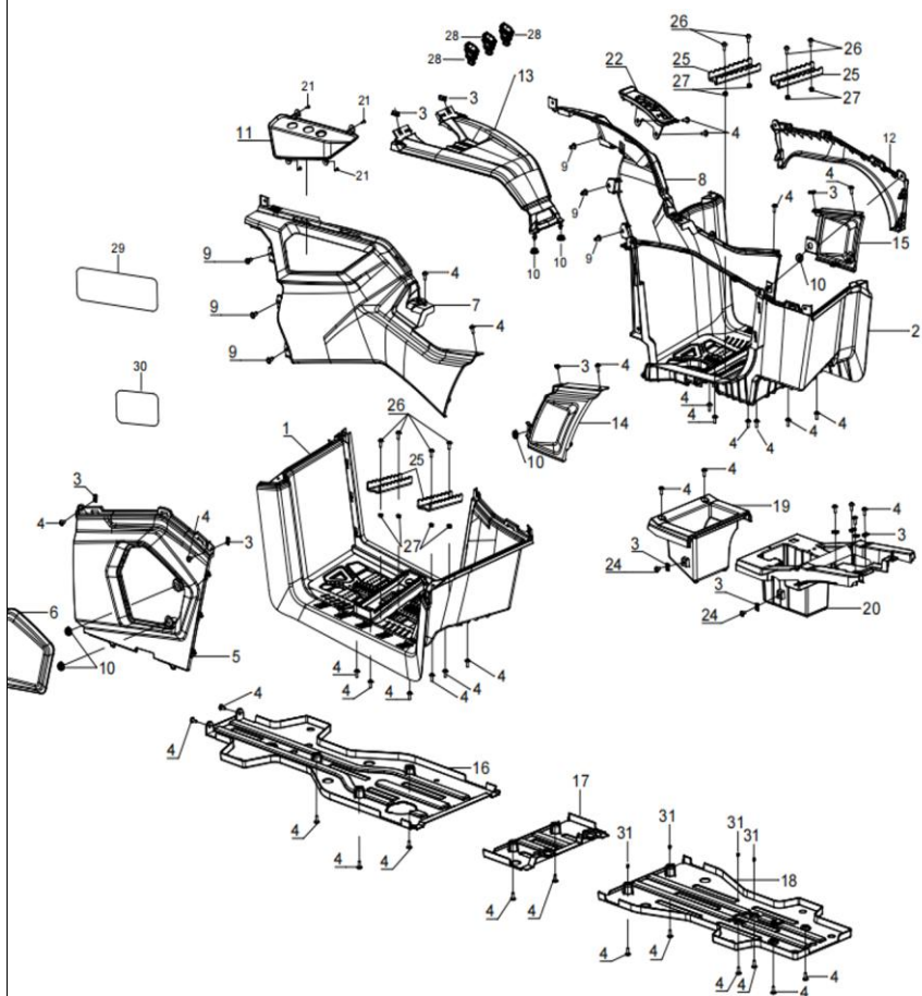
DIAGRAMMA 2025 PEDALE DEL PIEDE AODES F18
