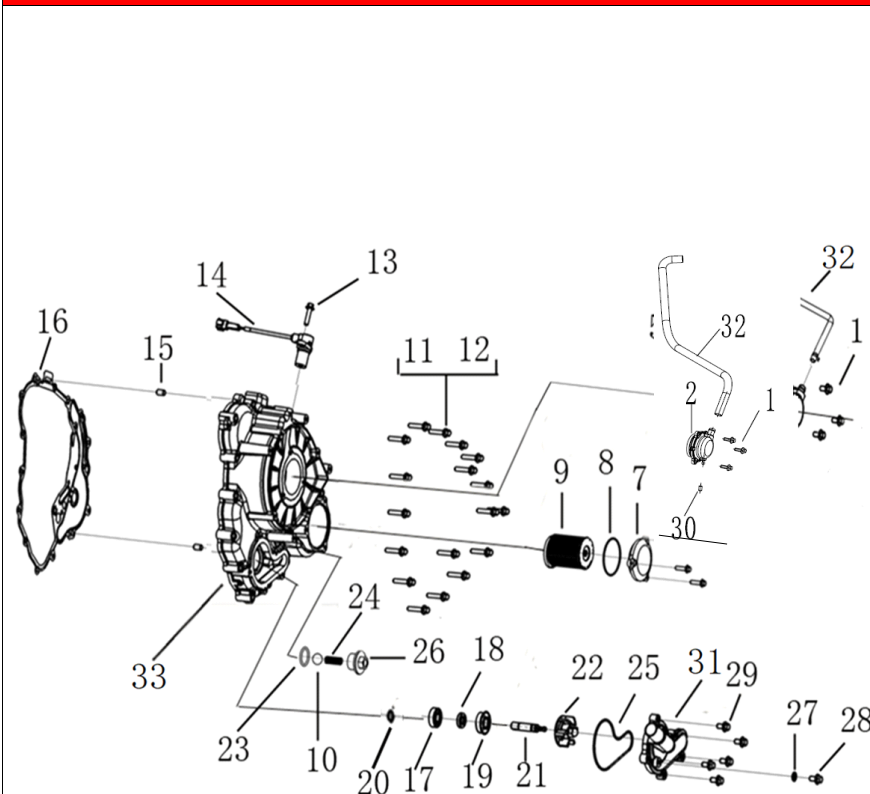
DIAGRAMMA 2025 COPERCHIO CARTER SINISTRO AODES E07
