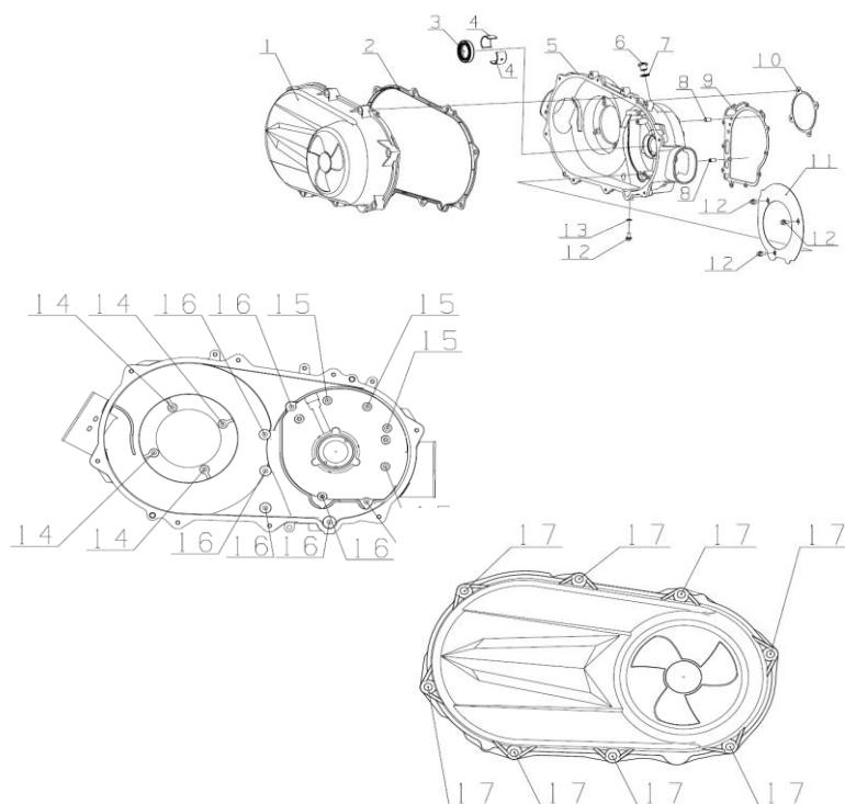
DIAGRAMMA 2025 COPERCHIO CARTER DESTRO AODES E04
