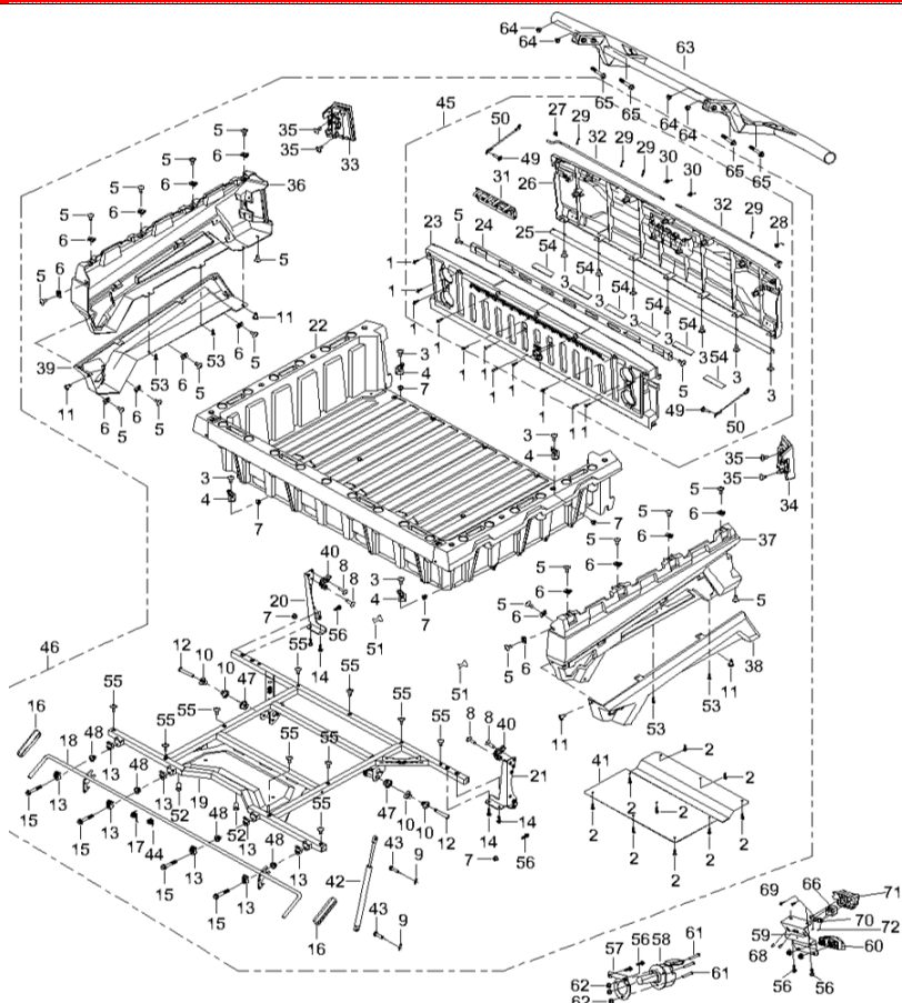
DIAGRAMMA 2025 CASSETTO PORTAOGGETTI AODES F23
