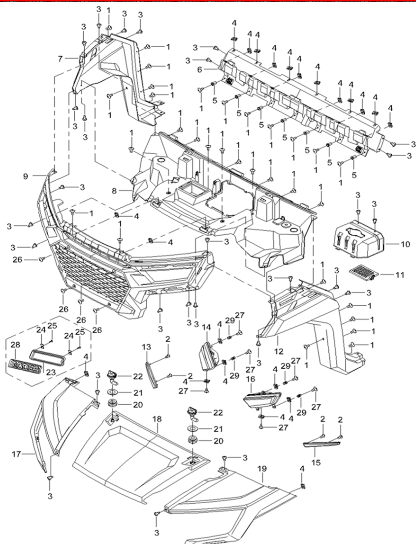
DIAGRAMMA 2025 PANNELLO ANTERIORE AODES F18
