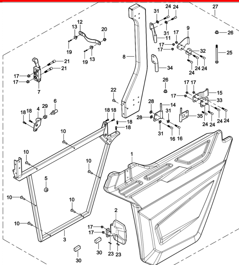
DIAGRAMMA 2025 PORTA ANTERIORE LATO GUIDA (QUATTRO PORTE) AODES F24
