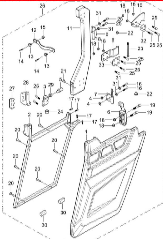
DIAGRAMMA 2025 PORTA POSTERIORE LATO GUIDA (QUATTRO PORTE) AODES F26
