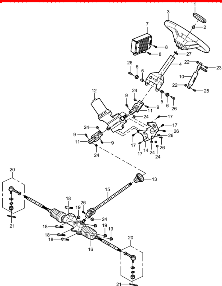
DIAGRAMMA 2025 SISTEMA STERZO AODES (CON EPS) F05
