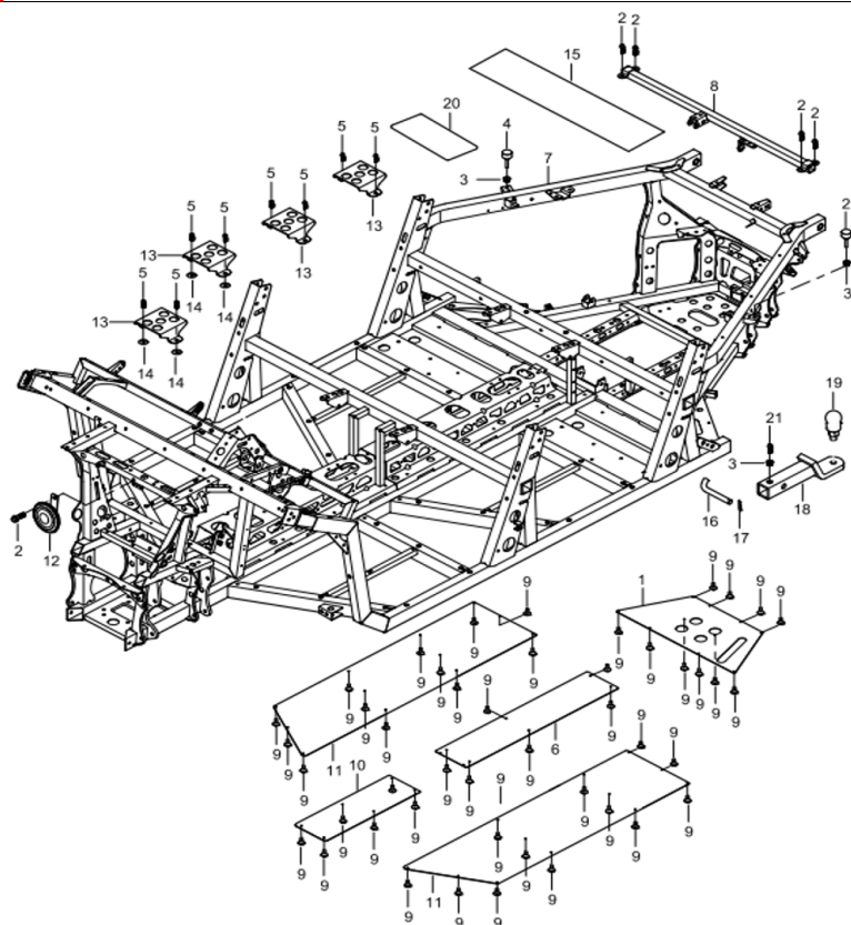
DIAGRAMMA 2025 TELAIO AODES (QUATTRO PORTE) F16
