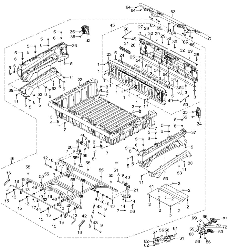
DIAGRAMMA 2025 SCATOLA PORTAOGGETTI AODES F23
