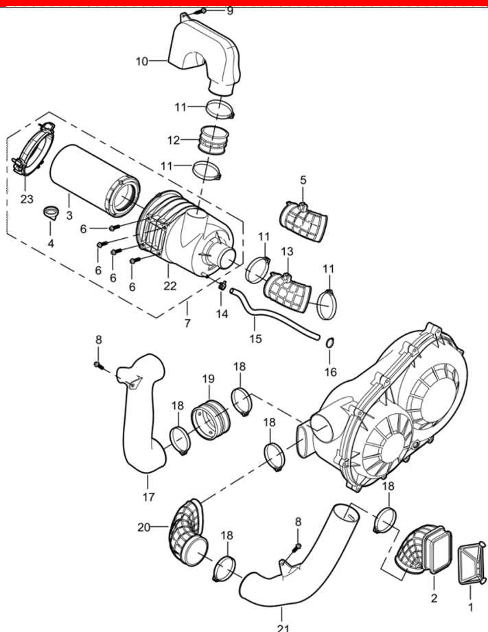
DIAGRAMMA 2025 SISTEMA FILTRO ARIA & INGRESSO & USCITA CVT AODES F10
