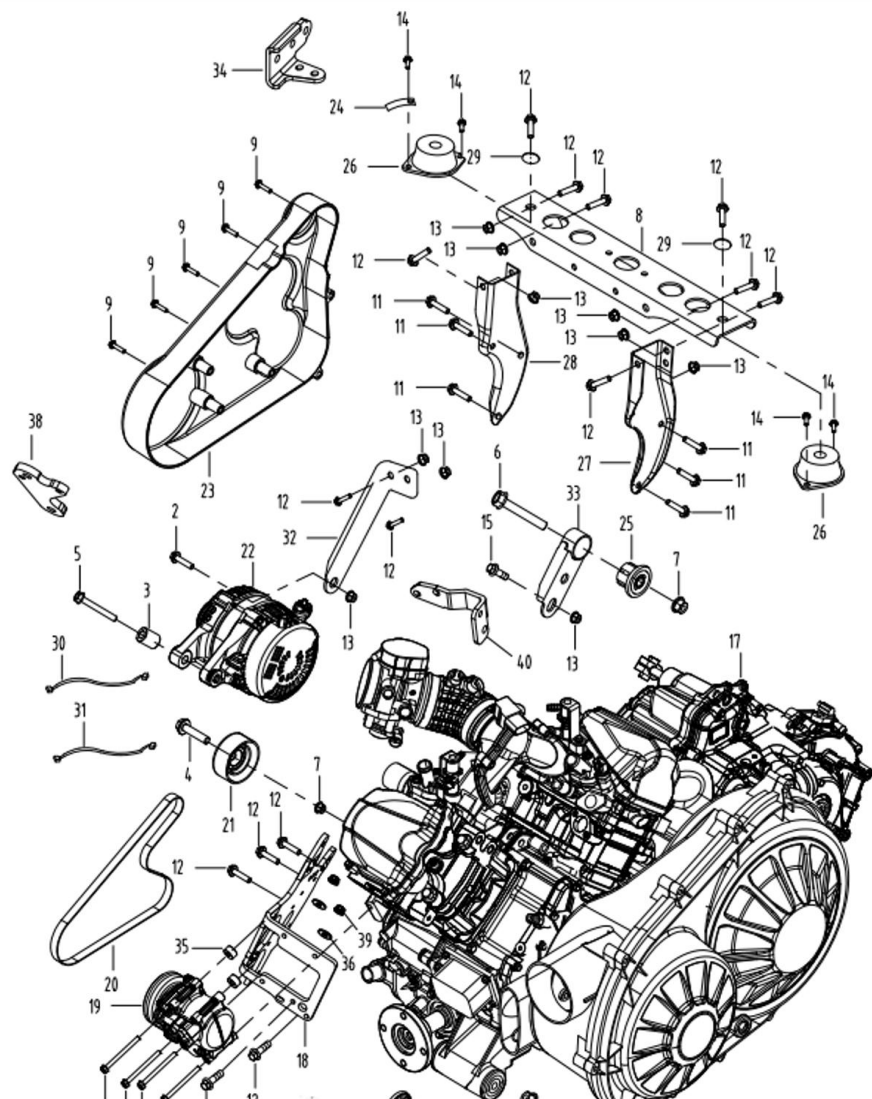
DIAGRAMMA 2025 MONTAGGIO MOTORE AODES F24
