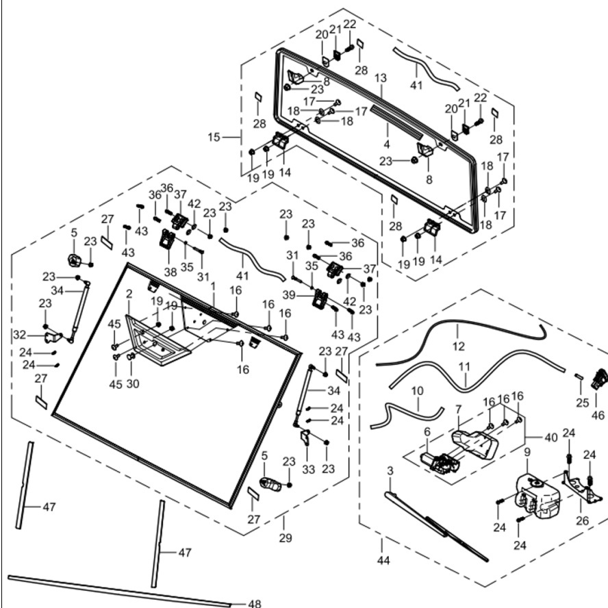
DIAGRAMMA 2025 FINESTRA ANTERIORE E POSTERIORE (OPZIONALE) AODES F11
