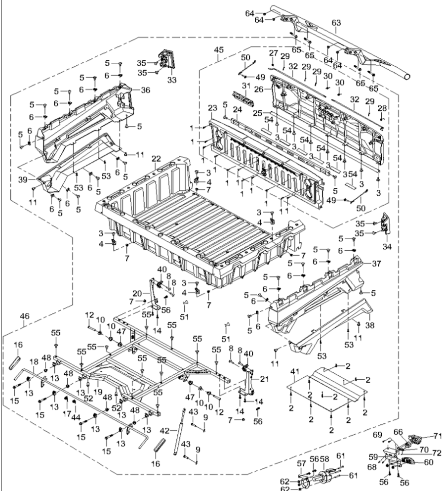
DIAGRAMMA 2025 SCATOLA PORTAOGGETTI AODES F23
