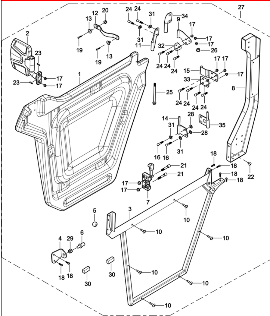
DIAGRAMMA 2025 PORTA ANTERIORE LATO PASSEGGERO (QUATTRO PORTE) AODES F25
