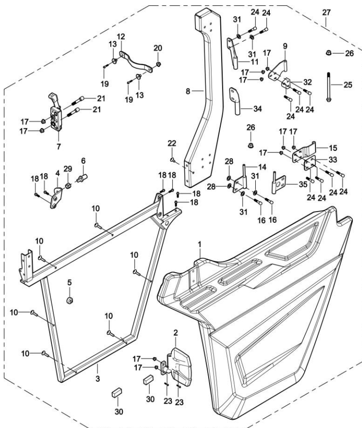
DIAGRAMMA 2025 PORTA ANTERIORE LATO GUIDA (QUATTRO PORTE) AODES F24
