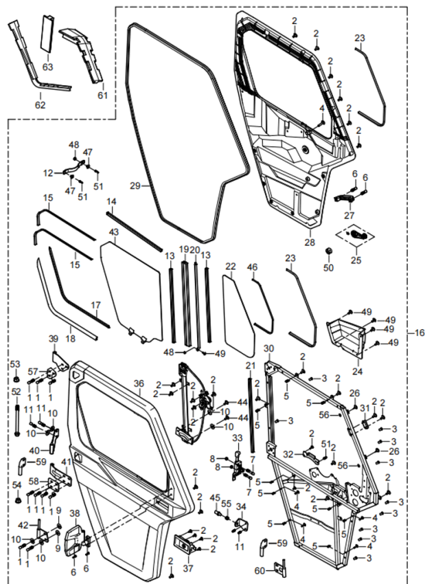
DIAGRAMMA 2025 PORTA ANTERIORE LATO PASSEGGERO (QUATTRO PORTE) AODES F21
