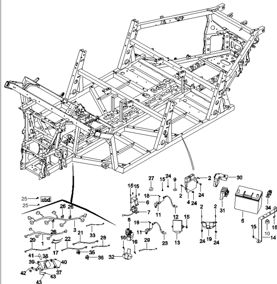
DIAGRAMMA 2025 COMPONENTI ELETTRICI AODES F22
