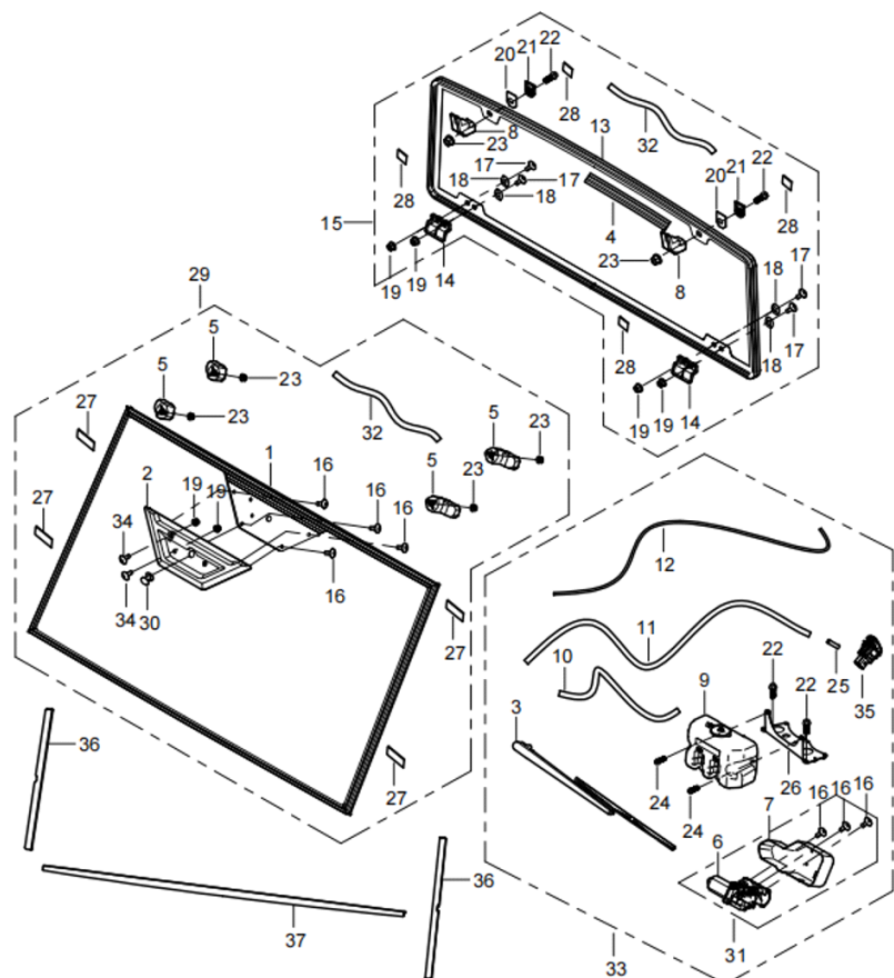
DIAGRAMMA 2025 FINESTRA ANTERIORE E POSTERIORE AODES F10
