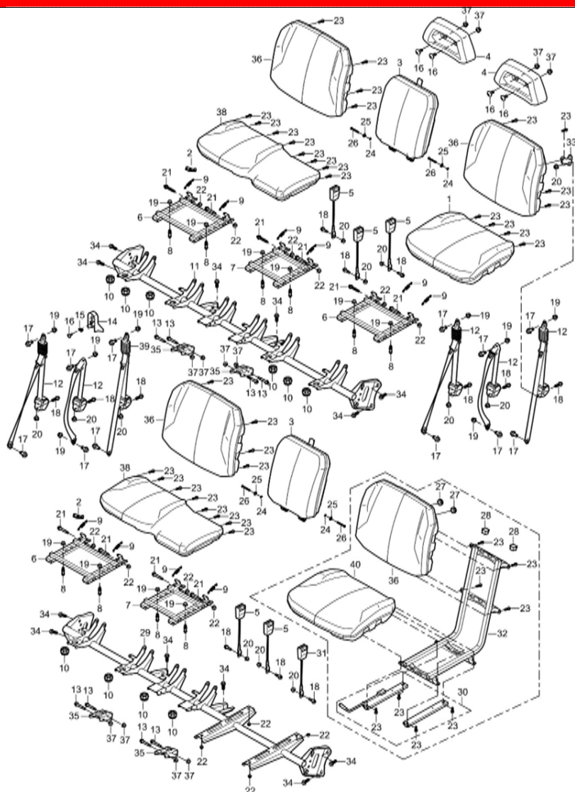
DIAGRAMMA 2025 SEDILI AODES (QUATTRO PORTE) F15
