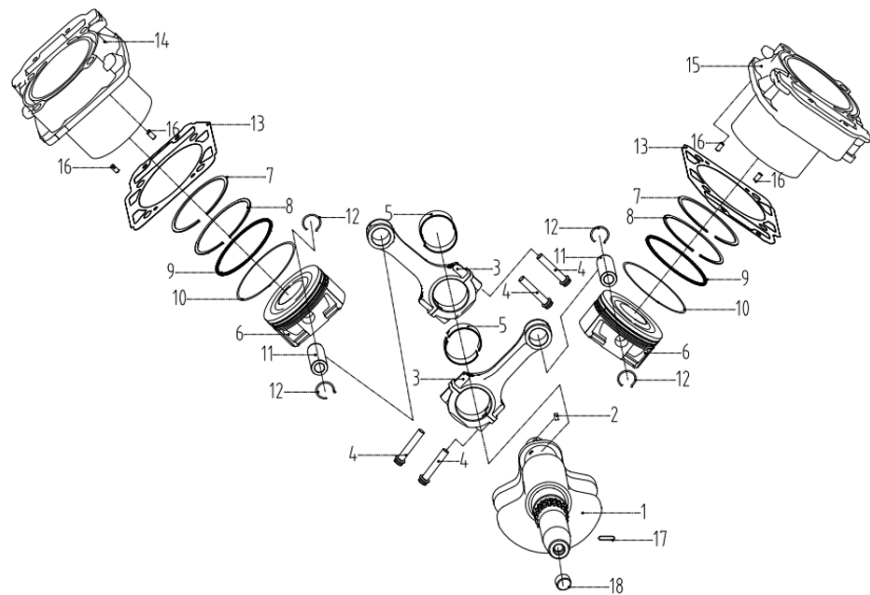
DIAGRAMMA 2025 ALBERO MOTORE, PISTONE E CILINDRO AODES E04
