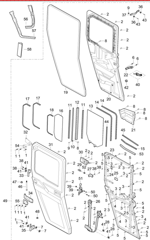
DIAGRAMMA 2025 PORTA POSTERIORE LATO PASSEGGERO (QUATTRO PORTE) AODES F23
