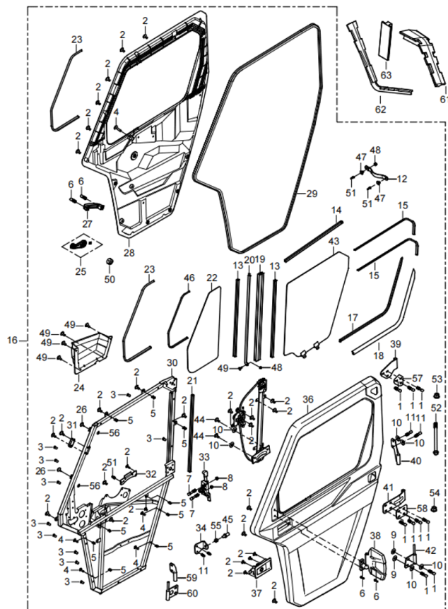
DIAGRAMMA 2025 PORTA ANTERIORE LATO GUIDA (QUATTRO PORTE) AODES F20
