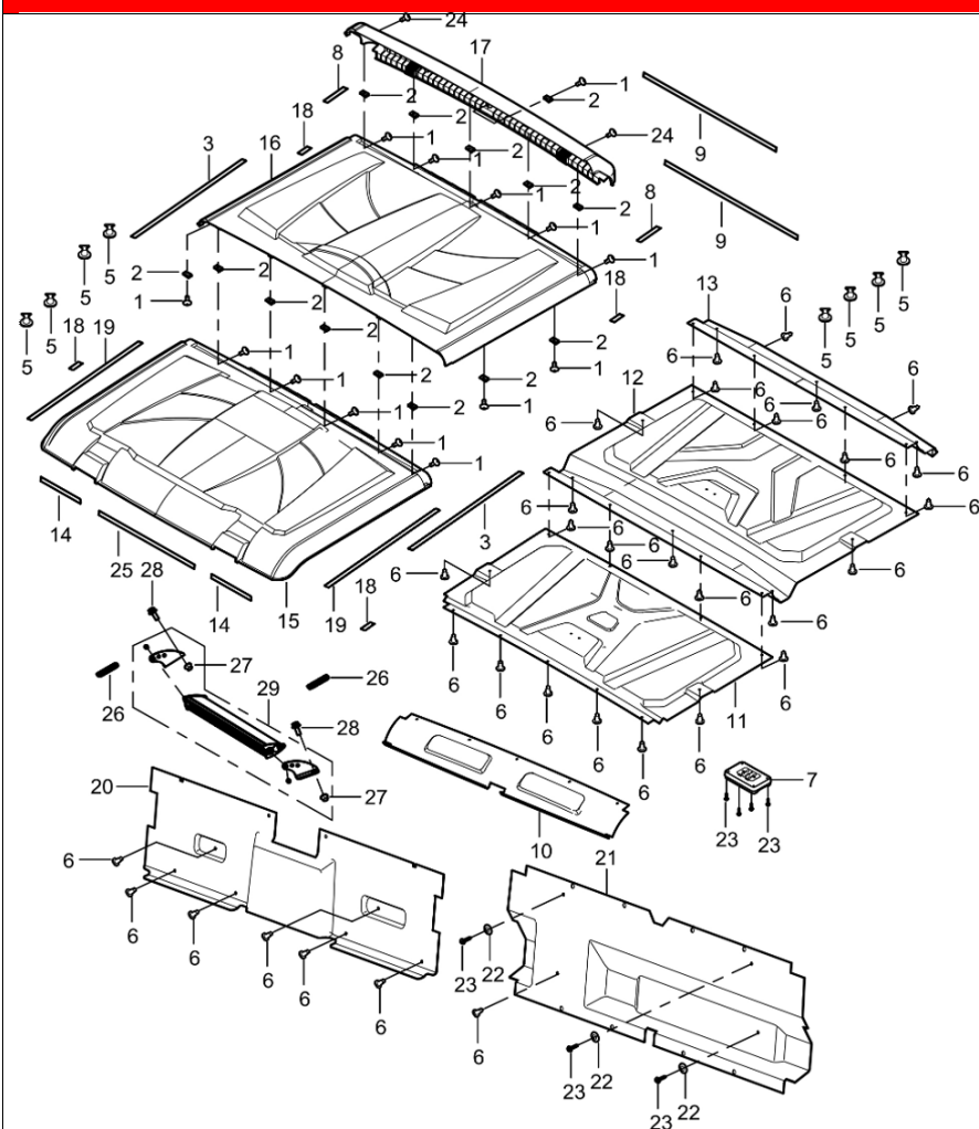
DIAGRAMMA 2025 TETTO AODES (QUATTRO PORTE) F13
