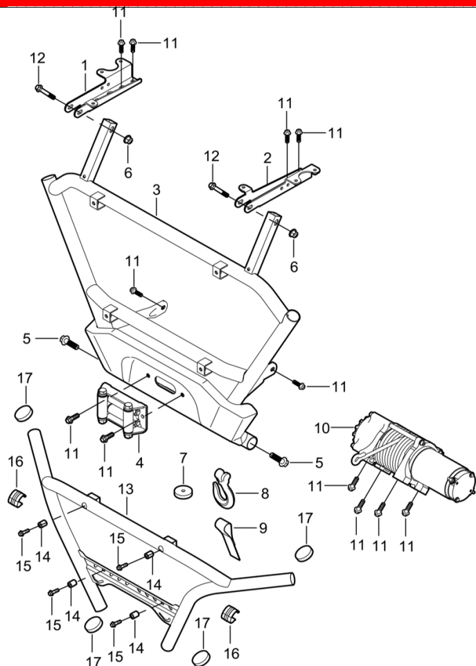
DIAGRAMMA 2025 VERRICELLO ANTERIORE E PARAURTI AODES F22
