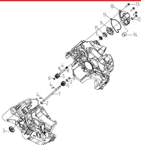
DIAGRAMMA 2025 RAFFREDDAMENTO MOTORE AODES E07
