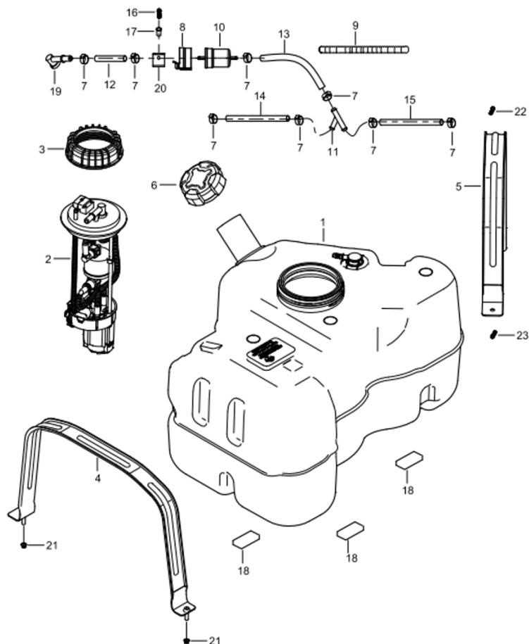
DIAGRAMMA 2025 SISTEMA CARBURANTE AODES F07
