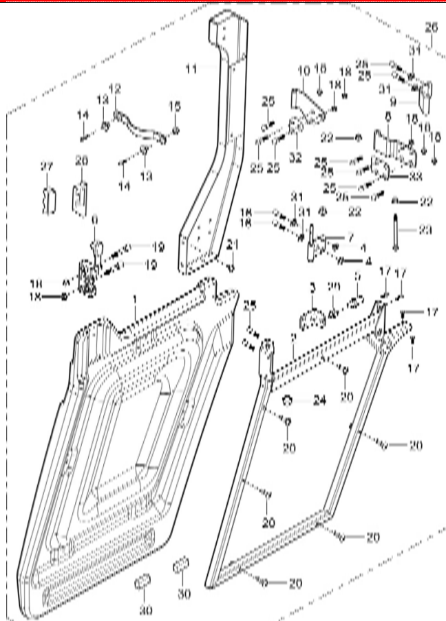
DIAGRAMMA 2025 PORTA ANTERIORE LATO PASSEGGERO (QUATTRO PORTE) AODES F27
