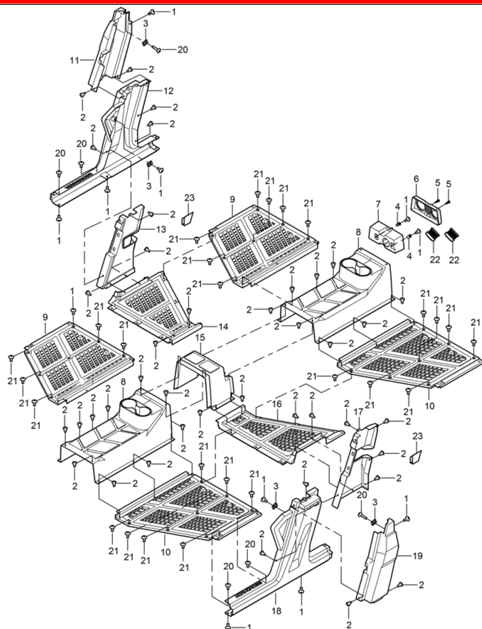
DIAGRAMMA 2025 PEDANA AODES (QUATTRO PORTE) F20
