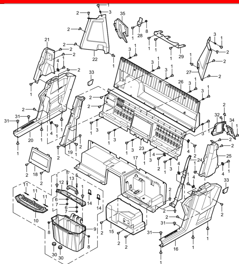
DIAGRAMMA 2025 PEDANA AODES (QUATTRO PORTE) F21
