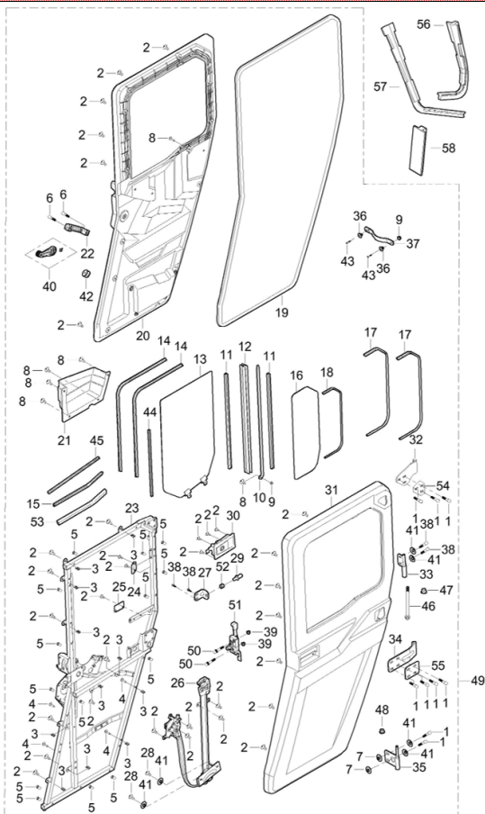
DIAGRAMMA 2025 PORTA POSTERIORE LATO GUIDA (QUATTRO PORTE) AODES F22
