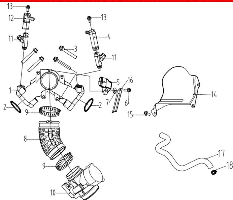
DIAGRAMMA 2025 MANIFOLDO DI INGRESSO E CORPO FARFALLATO AODES E09
