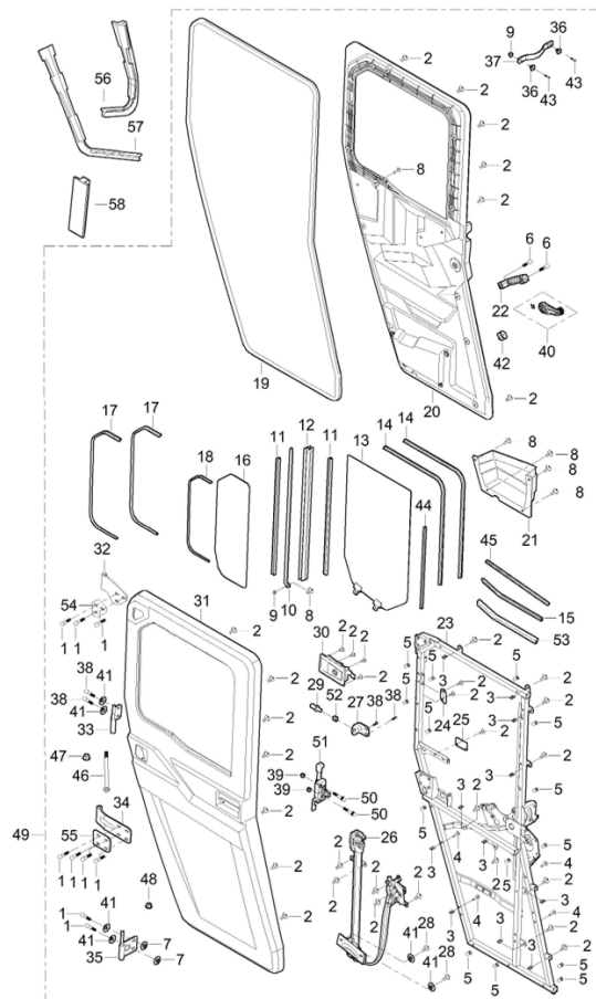
DIAGRAMMA 2025 PORTA POSTERIORE LATO PASSEGGERO (QUATTRO PORTE) AODES F23
